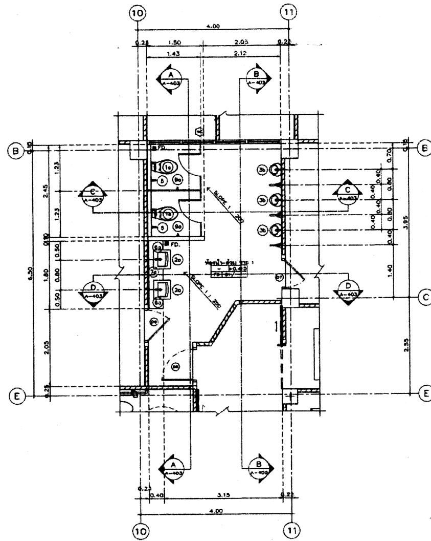
แปลนพื้นที่ห้องน้ำ - ส่วน ชาย 1 มาตราส่วน 1:50
